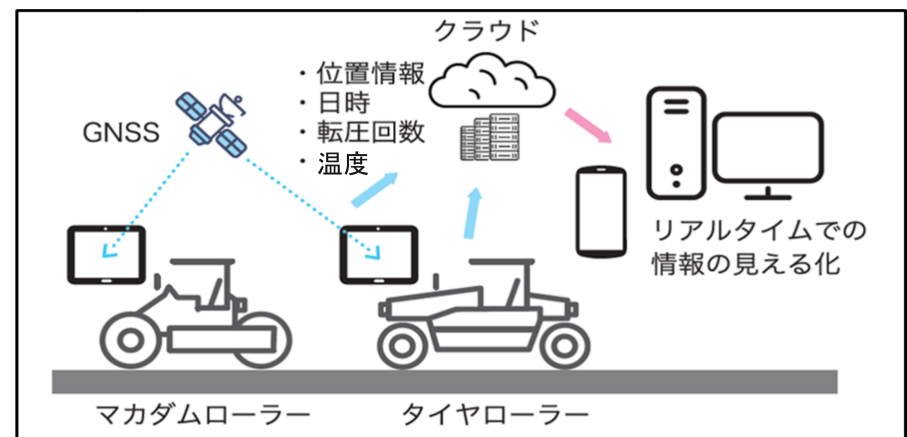
転圧温度管理モニター
